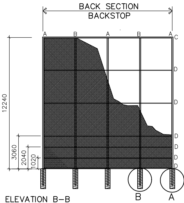
ELEVATION A-A
